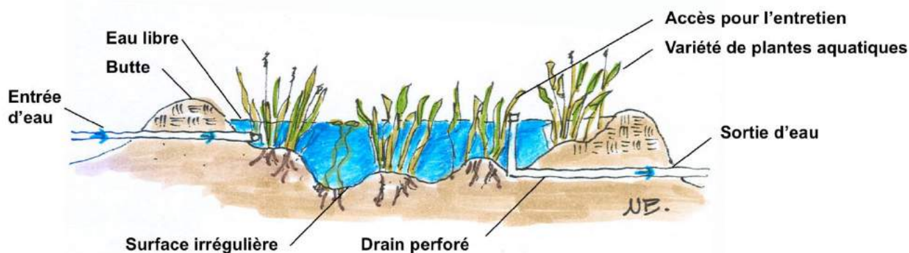
Figure 12. Marais filtrant à écoulement des eaux sur la surface. Illustration : N. Bédard
