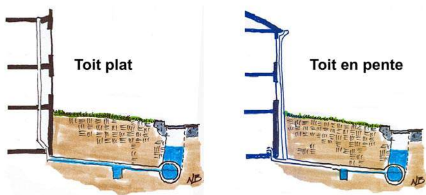
Figure 6. Connexions conventionnelles des gouttières. Illustration : N. Bédard
