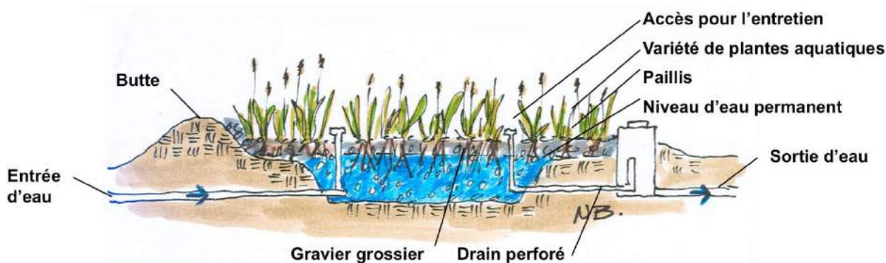
Figure 13. Marais filtrant à écoulement des eaux sous la surface. Illustration : N. Bédard
