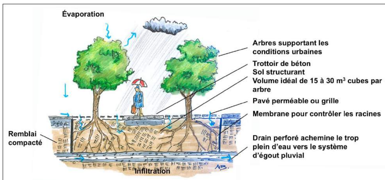
Figure 10. Fosse de plantation d'arbres en continu. Illustration: N. Bédard
