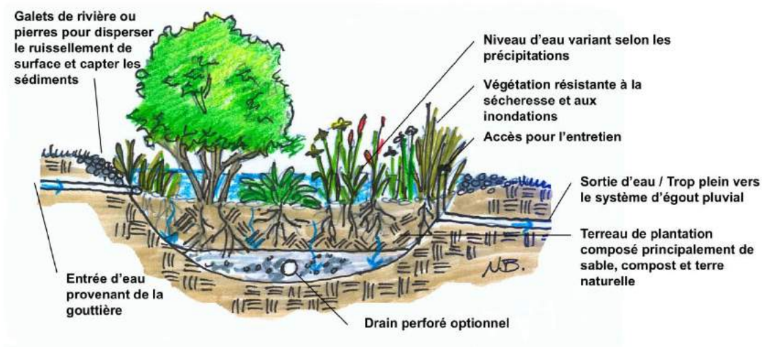
Figure 8. Jardin de pluie. Illustration : N. Bédard
