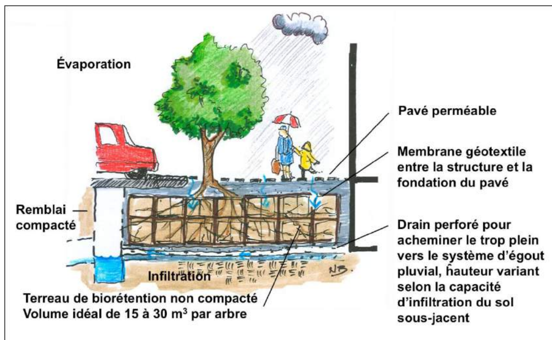
Figure 11. Fosse de plantation d'arbres avec structure souterraine. Illustration : N. Bédard
