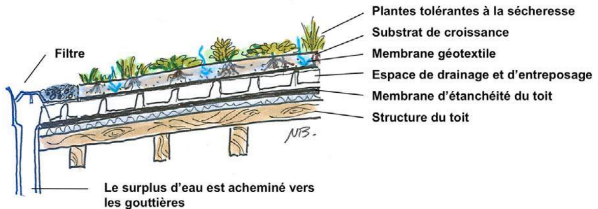
Figure 5. Toit vert extensif. Illustration : N. Bédard
